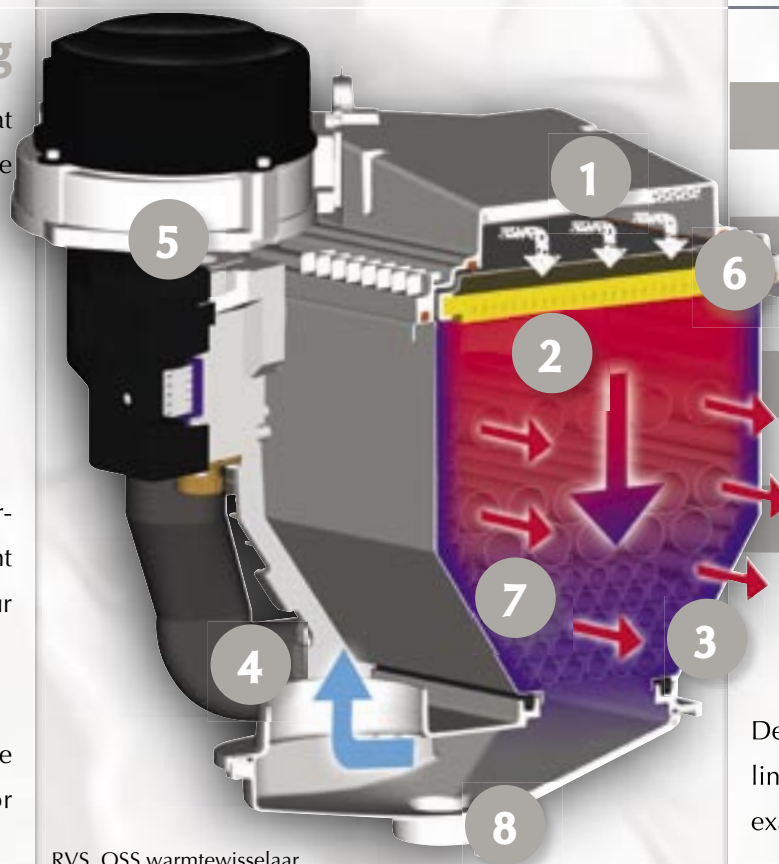
RVS OSS warmtewisselaar
